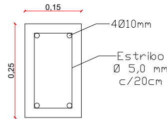
VIGA INFERIOR + VIGA SUPERIOR (MUROS) Escala 1/50
