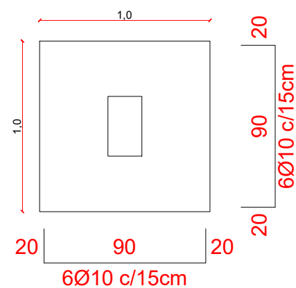
SAPATAS (P1 a P4) - MUROS Escala 1/50
