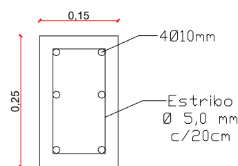
PILARES MUROS Escala 1/50
