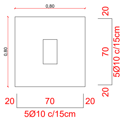
SAPATAS (P5 a P8) - MUROS Escala 1/50
